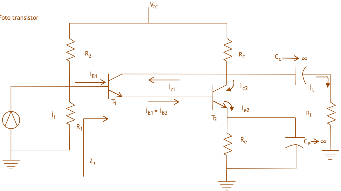
Fotodiodo a amplificador FET
